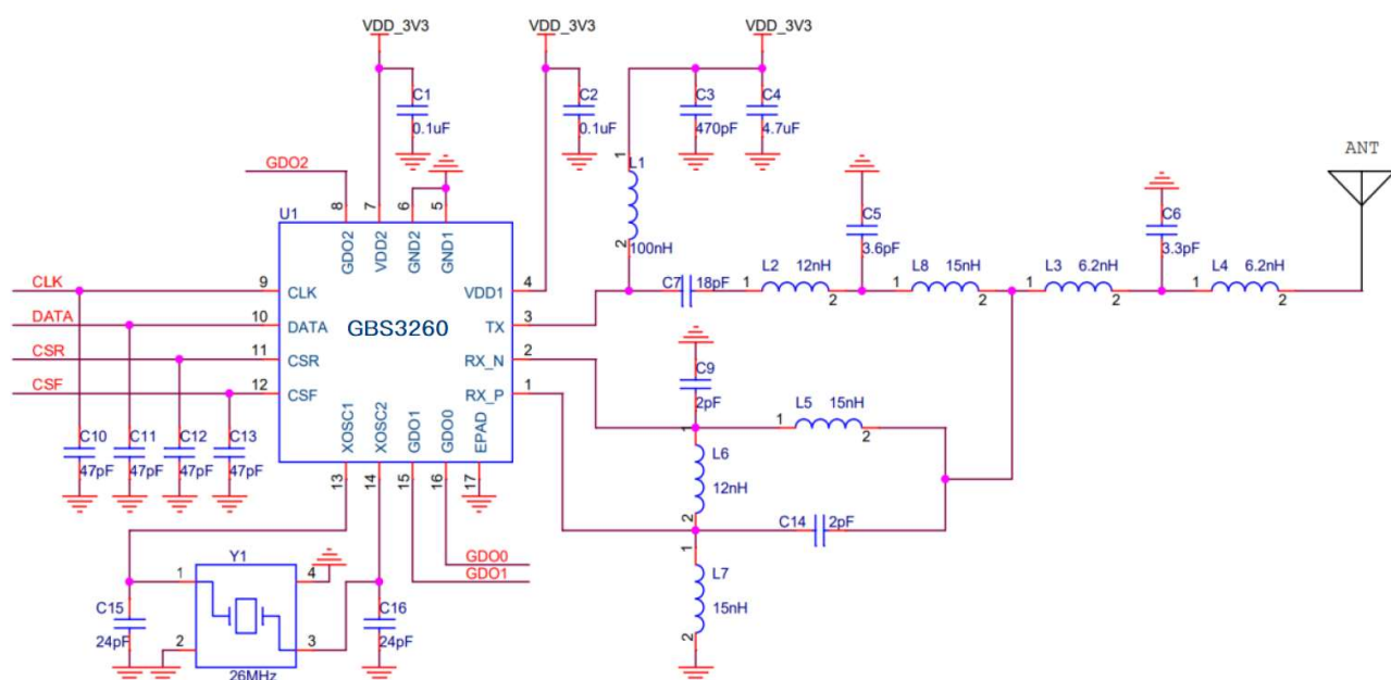
图 13 GBS3260-868MHz-Direct-20dBm 典型应用
