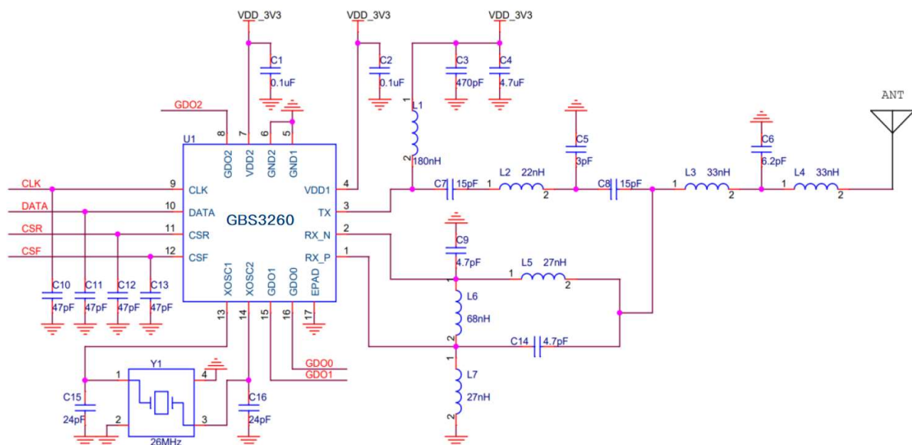
图 12 GBS3260-433MHz-Direct-20dBm 典型应用
