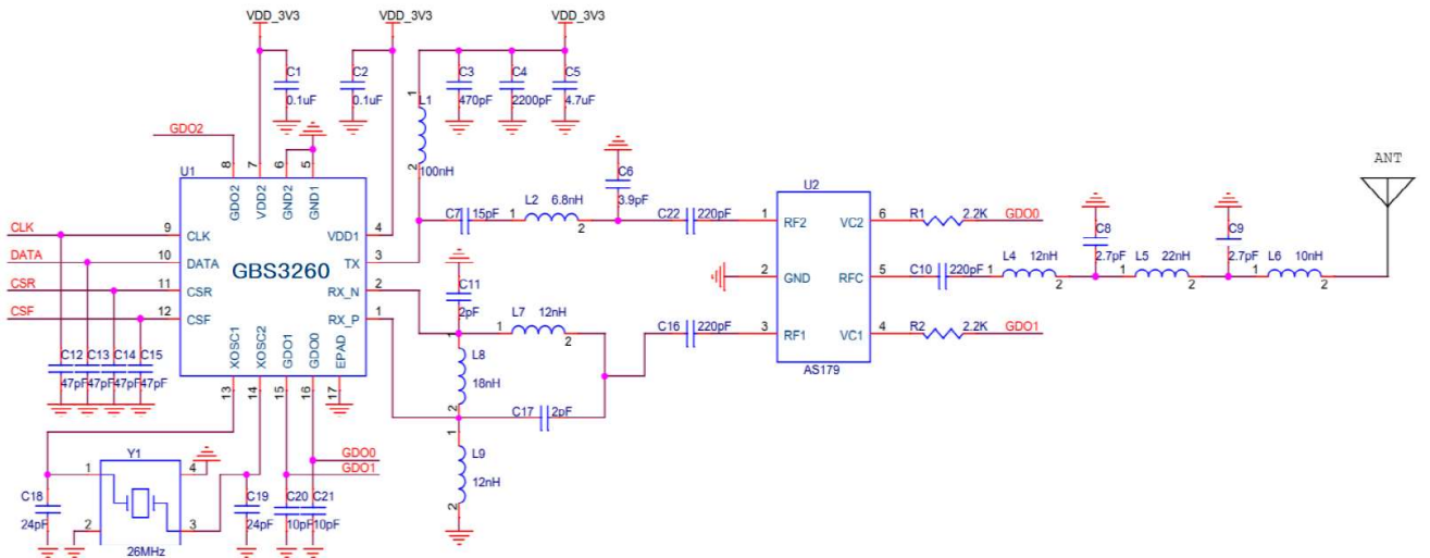
图 15 GBS3260-868MHz-SPDT-20dBm 典型应用
