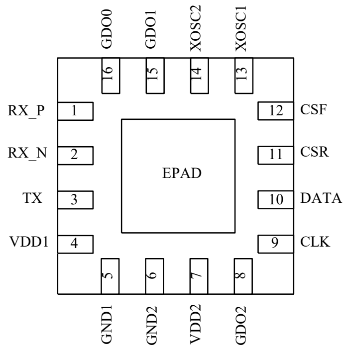
图 2 GBS3260 管脚排列图
