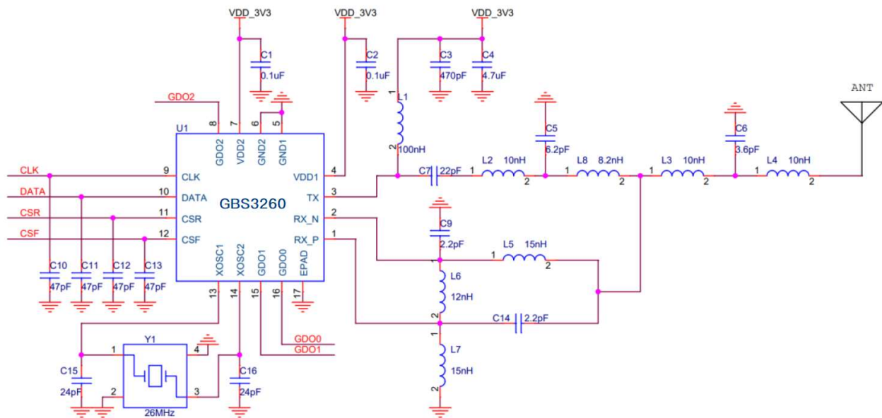
图 11 GBS3260-868MHz-Direct-13dBm 典型应用
