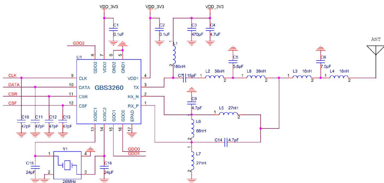
图 10 GBS3260-433MHz-Direct-13dBm 典型应用
