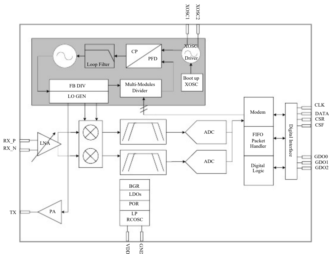
图 3 GBS3260 系统框图
